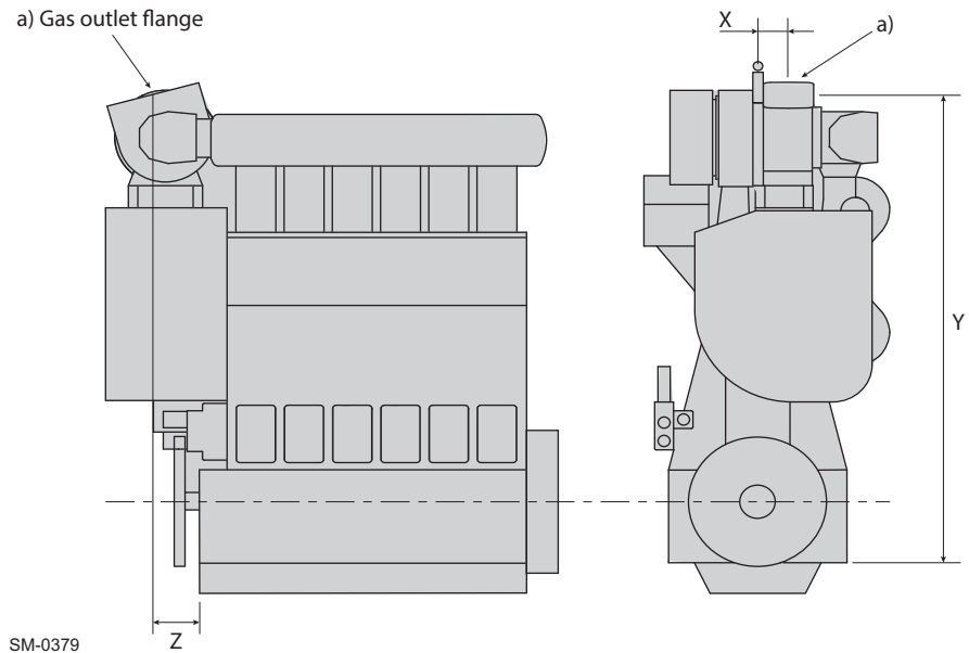
Figure 3-2 Thermal expansion, dim. X, Y, Z
