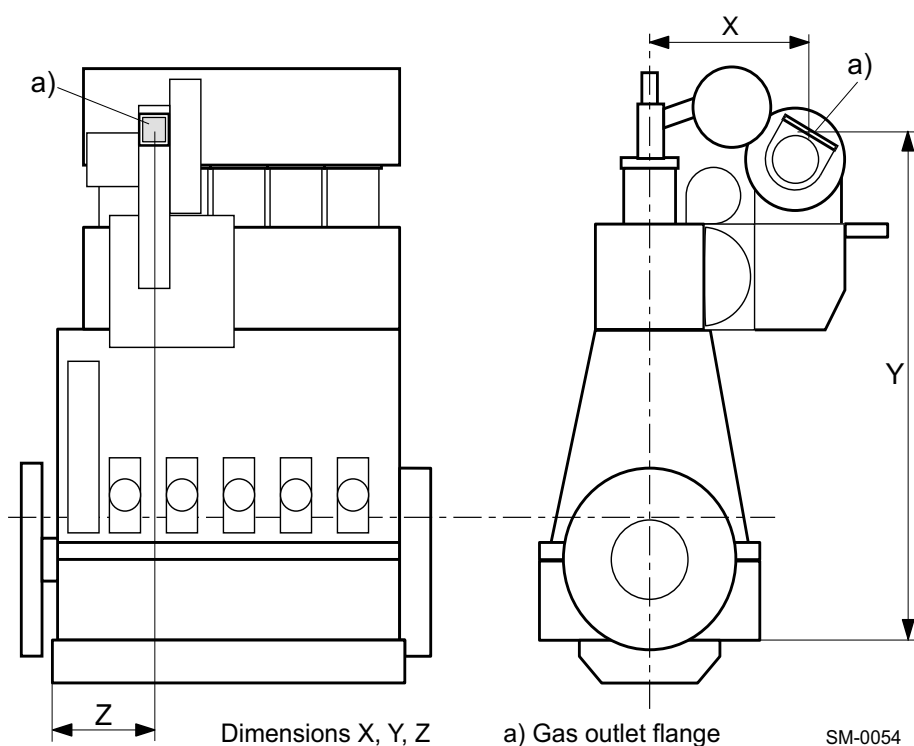
Figure 3-2 Thermal expansion, dim. X, Y, Z
